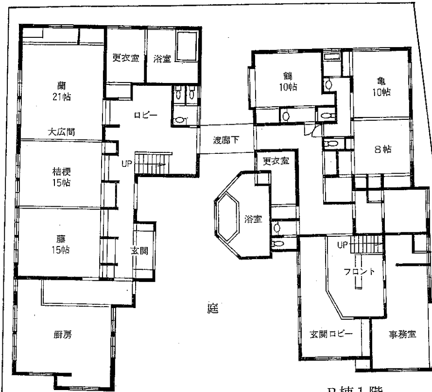
A棟1階
